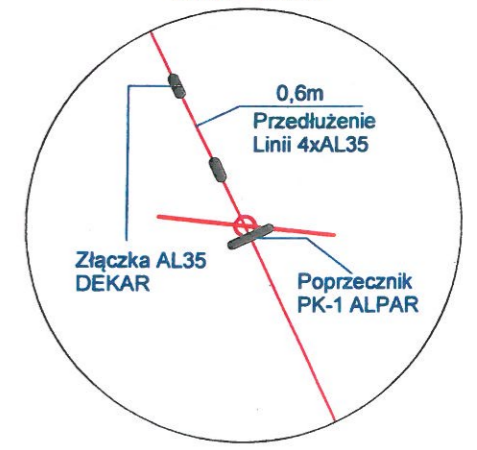
Słup nr 11 Skala 1:10
